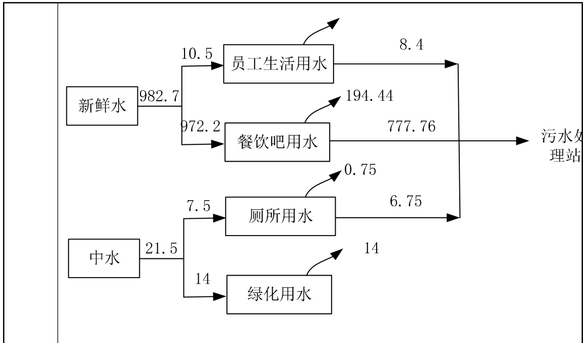
图 2-1 水平衡图 (单位 m 3 /d)
